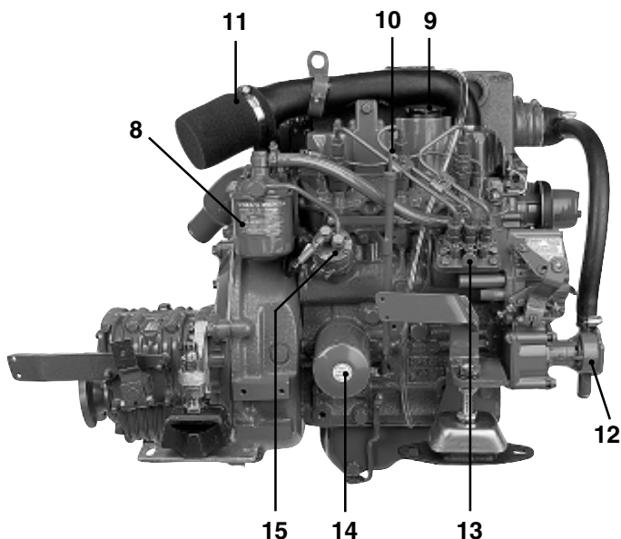
MD2030 med backslag MS10A
